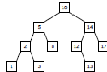
Binärer Suchbaum
